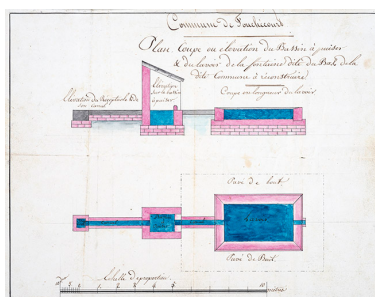
Plan et coupe de la fontaine du bas du village à reconstruire (1861). Phot. Jérôme Mongreville, Autr. Servas IVR43_20167000941NUC4A
