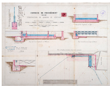
Projet de construction de bassins (1871). Phot. Jérôme Mongreville, Autr. Jacques Humbert IVR43_20167000945NUC4A
