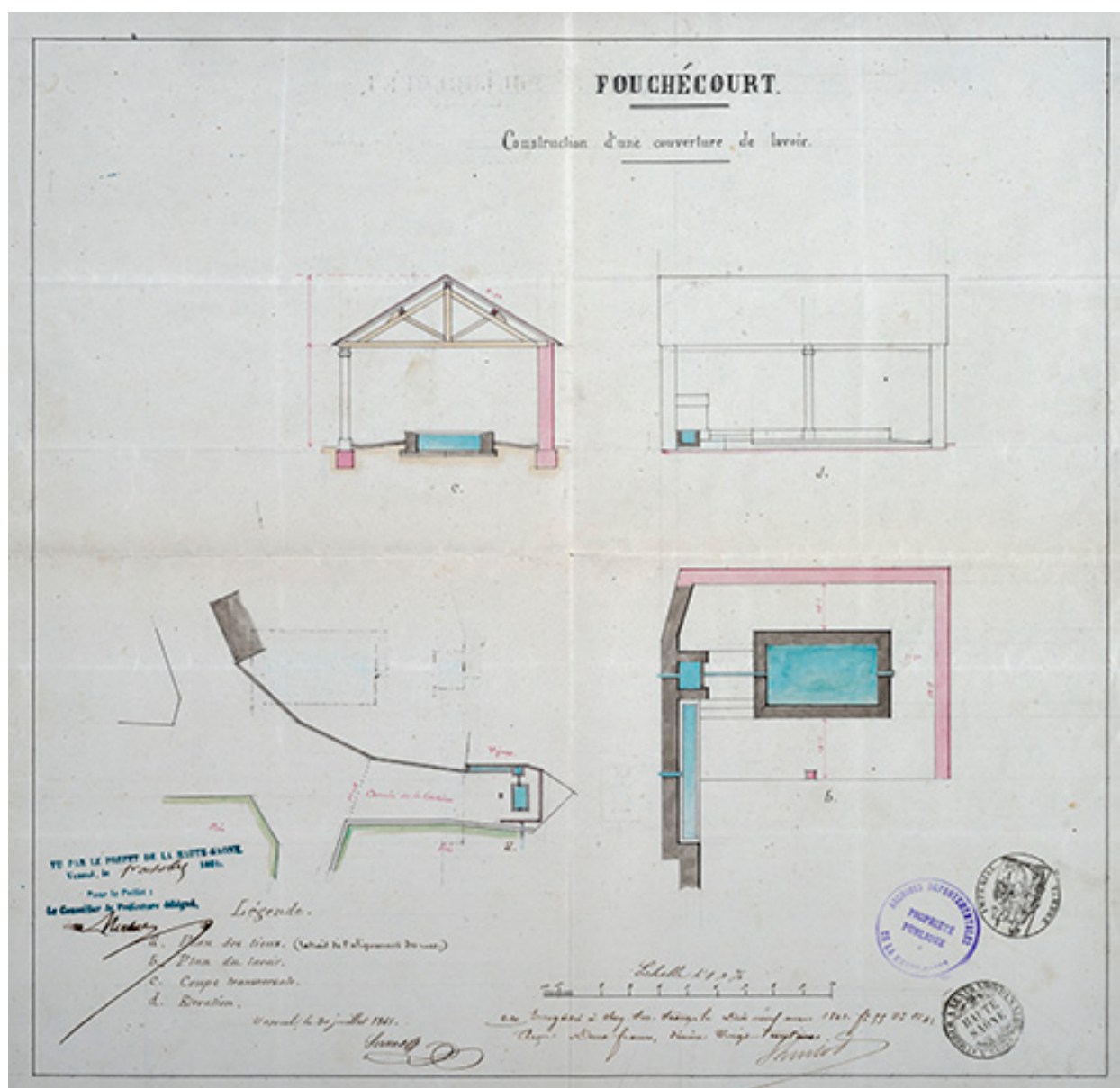
Projet de couverture d'un lavoir (1861).
