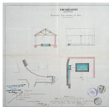
Projet de couverture d'un lavoir (1861). Phot. Jérôme Mongreville, Autr. Servas IVR43_20167000947NUC4A
