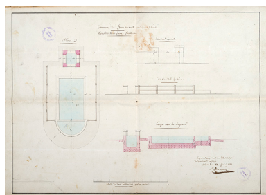
Projet pour la construction d'un lavoir (1828). Phot. Jérôme Mongreville, Autr. Moreau IVR43_20167000951NUC4A
