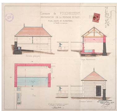
Restauration de la fontaine du "haut" (1901). Phot. Jérôme Mongreville, Autr. Jacques Humbert IVR43_20167000943NUC4A
