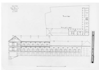
Projet de François Agnétty présenté au Conseil des Bâtiments civils en septembre 1836, élévation et plan du second étage.
