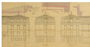
Projet de pavillon annexe, par l'architecte René Moreau (11 janvier 1897), façades. Repro. Pierre-Marie Barbe- Richaud, Autr. René Moreau IVR26_20217100344NUC2A
