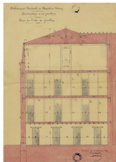
Projet de pavillon annexe, par l'architecte René Moreau (11 janvier 1897), coupe. Repro. Pierre-Marie Barbe- Richaud, Autr. René Moreau IVR26_20217100343NUC2A
