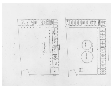
Projet de François Agnétty présenté au Conseil des Bâtiments civils en septembre 1836, plan du rez-de-chaussée et plan du premier étage.
