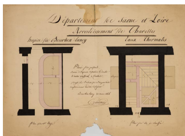
Projet pour la construction d'un bain de vapeur, plan du rez-de-chaussée et de l'étage (1846).
