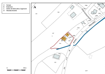
Plan-masse et de situation. Extrait du plan cadastral, 2017, section B, 1/2 500 agrandi à 1/1 000. Dess. Bertrand Turina IVR43_20182501325NUDA
