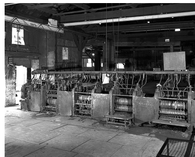
Laminage vu de trois quarts droit. Phot. Yves Sancey IVR43_19923900896X
