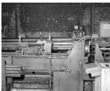
Banc d'étirage : étirage. Phot. Yves Sancey IVR43_19923900914X
