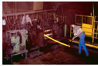
Laminage : travail en cage de dégrossis. Phot. Yves Sancey IVR43_19943900033ZA
