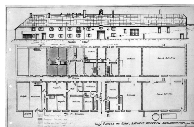
Forges de Syam. Bâtiment direction-administration. Phot. Jérôme Mongreville IVR43_19923900834V
