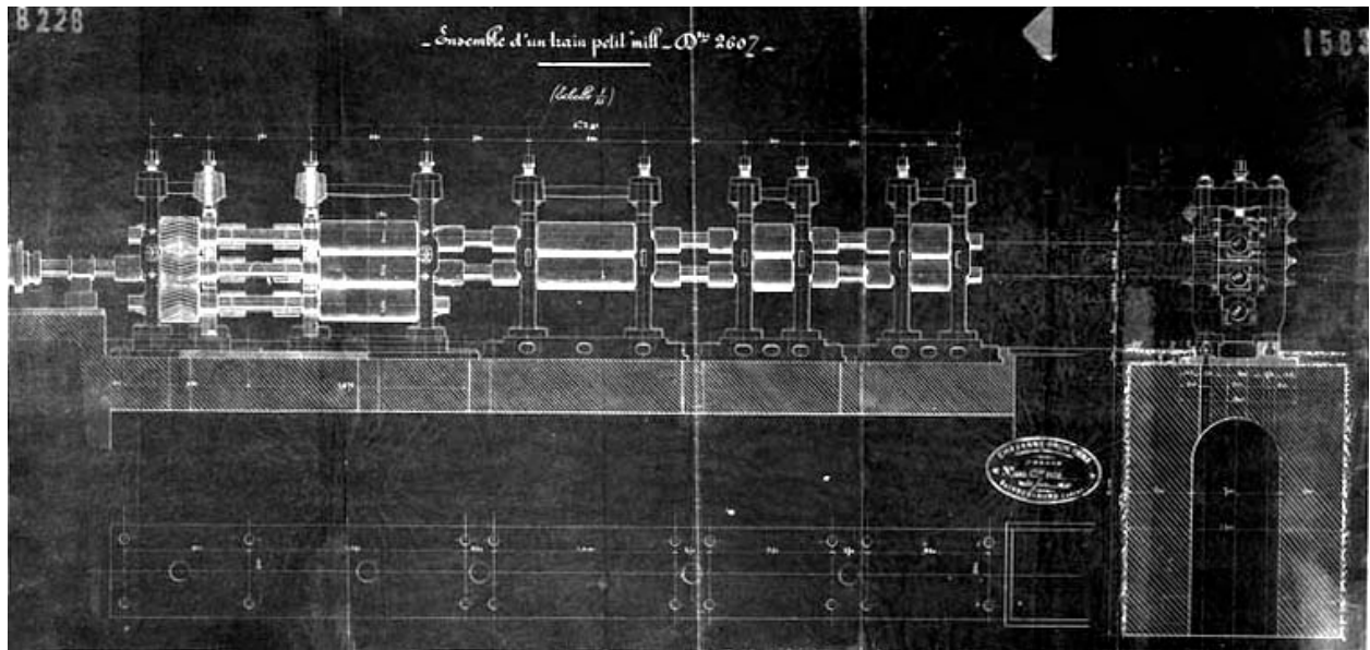
Ensemble d'un train petit mill. Dtre 260 m/m.
