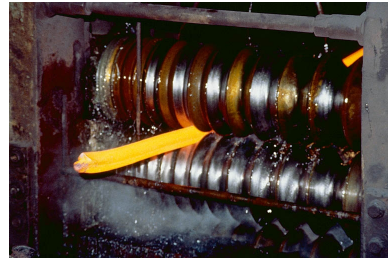
Laminage : travail en cage de dégrossis (détail). Phot. Yves Sancey IVR43_19943900050ZA
