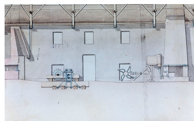
Coupe sur la longueur de la forge [détail de la refenderie, du laminoir et du soufflet]. Phot. Daniel Lebée IVR43_19933900046XA
