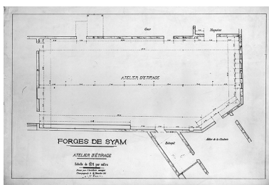
Forges de Syam. Atelier d'étrirage. Phot. Jérôme Mongreville, Phot. Charles-Alfred Schacre IVR43_19923900827V
