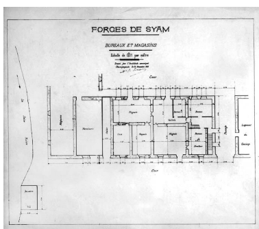
Forges de Syam. Bureaux et magasins. Phot. Jérôme Mongreville, Phot. Charles-Alfred Schacre IVR43_19923900823V
