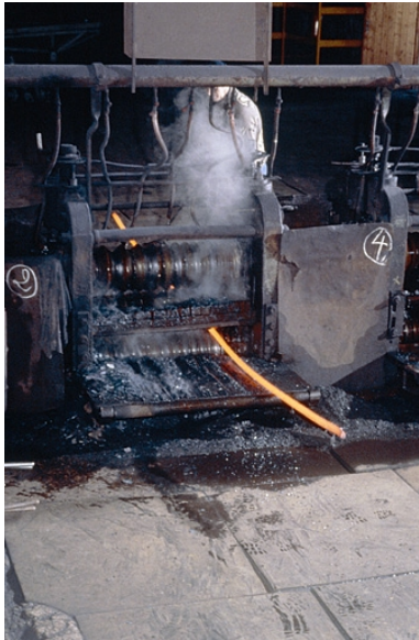
Laminage : travail en cage de dégrossis (détail). Phot. Yves Sancey IVR43_19943900059ZA
