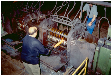
Laminage : travail en cage de dégrossis. Phot. Yves Sancey IVR43_19943900046ZA
