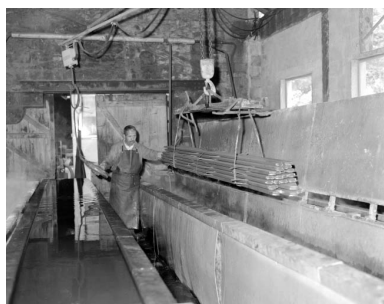
Atelier de décapage : déplacement des barres. Phot. Yves Sancey IVR43_19923900976X
