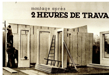
Montage d'une maison tout acier dans les années 1930 : mise en place des murs. Phot. Yves Sancey IVR43_19943900836ZA
