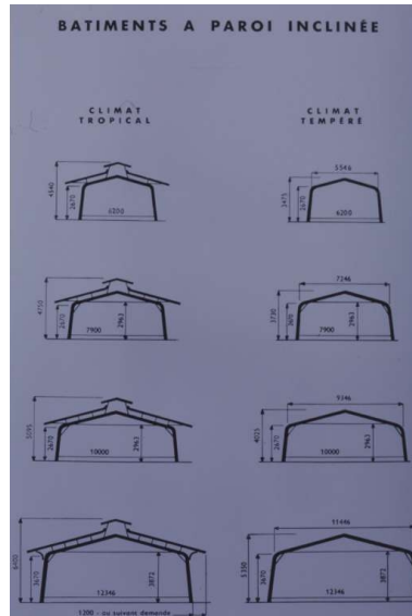
Bâtiments à paroi inclinée au début des années 1960 [modèles vus en coupe]. Phot. Jérôme Mongreville IVR43_19973901147ZA
