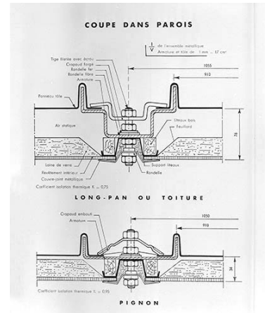
[Bâtiment à paroi inclinée au début des années 1960 : ] Coupe dans parois. Phot. Jérôme Mongreville IVR43_19963900092X
