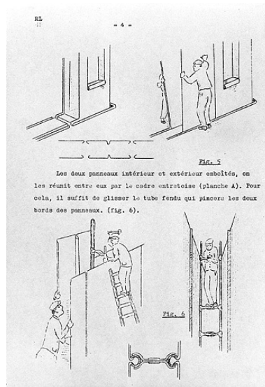
Schémas de montage des murs d'une maison tout acier. Phot. Yves Sancey IVR43_19943900843X
