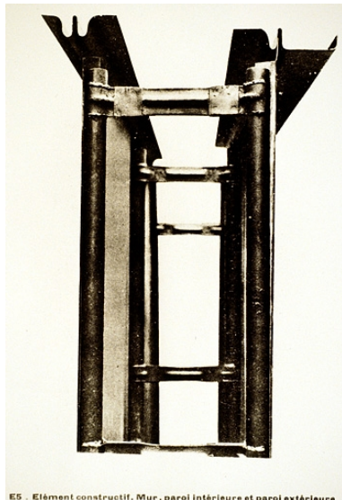
Elément constructif. Mur, paroi intérieure et paroi extérieure, 1929. Phot. Yves Sancey IVR43_19943900841ZA
