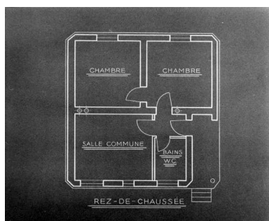
Exemple de construction dans les années 1930 : plan d'une maison T4 à usage de conciergerie. Phot. Yves Sancey IVR43_19943900013X
