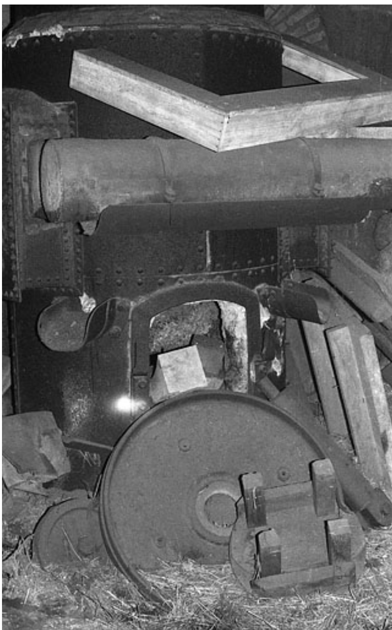
Base du petit coulée cubilot (3,5 tonnes).
