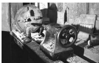
Vue rapprochée du tour horizontal. Phot. Rémi Hamelin IVR43_20107000037NUC2A
