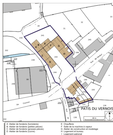
Plan-masse et de situation. Extrait du plan cadastral numérisé, 2008, section AR, 1:1000. Source : Direction générale des Finances Publiques - Cadastre ; mise à jour : 2008. Dess. André Céréza IVR43_20087001010NUDA
