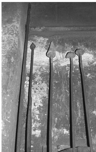
Ringards (bouchage et débouchage du trou de coulée). Phot. Rémi Hamelin IVR43_20107000044NUC2A
