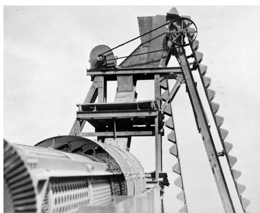
Le trommel, 1931. Phot. Yves Sancey IVR43_19893900018X
