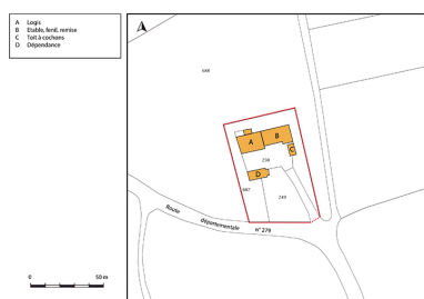
Plan-masse et de situation. Extrait du plan cadastral, 2018, section A, Echelle 1/1000. Dess. Bertrand Turina
