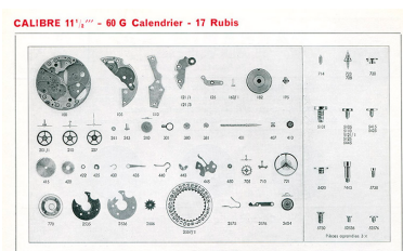
Calibre 11 1/2''' - 60 G Calendrier - 17 rubis [éclaté des fournitures du Parrenin HP 60 G], 1973. IVR43_20162500632NUC4A
