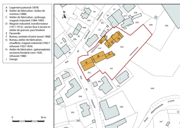
Plan-masse et de situation, avec datation. Extrait du plan cadastral, 2012, section AD. Dess. Mathias Papigny IVR43_20142501508NUDA
