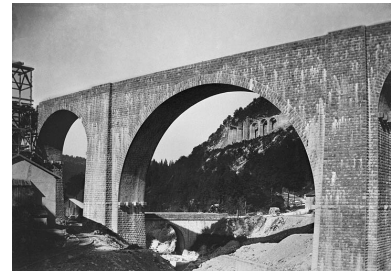
Travaux du chemin de fer : l'aqueduc [viaduc] de l'Evalude et le viaduc des Crottes, 1899. Phot. Jérôme Mongreville, Autr. Luc Paget IVR43_19913900055X
