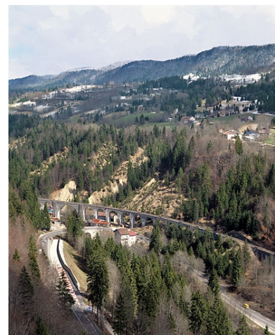
Vue d'ensemble plongeante, depuis l'ouest. Phot. Yves Sancey IVR43_20053900399XA
