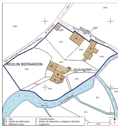
Plan-masse et de situation. Extrait du plan cadastral numérisé, 2008, section B, 1:1000. Source : Direction générale des Finances Publiques - Cadastre ; mise à jour : 2008. Dess. André Céréza
