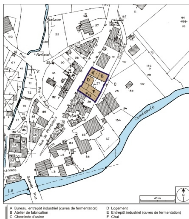
Plan-masse et de situation. Extrait du plan cadastral numérisé, 2008, section AC, 1:1000 réduit à 1:1250. Source : Direction générale des Finances Publiques - Cadastre ; mise à jour : 2008.
