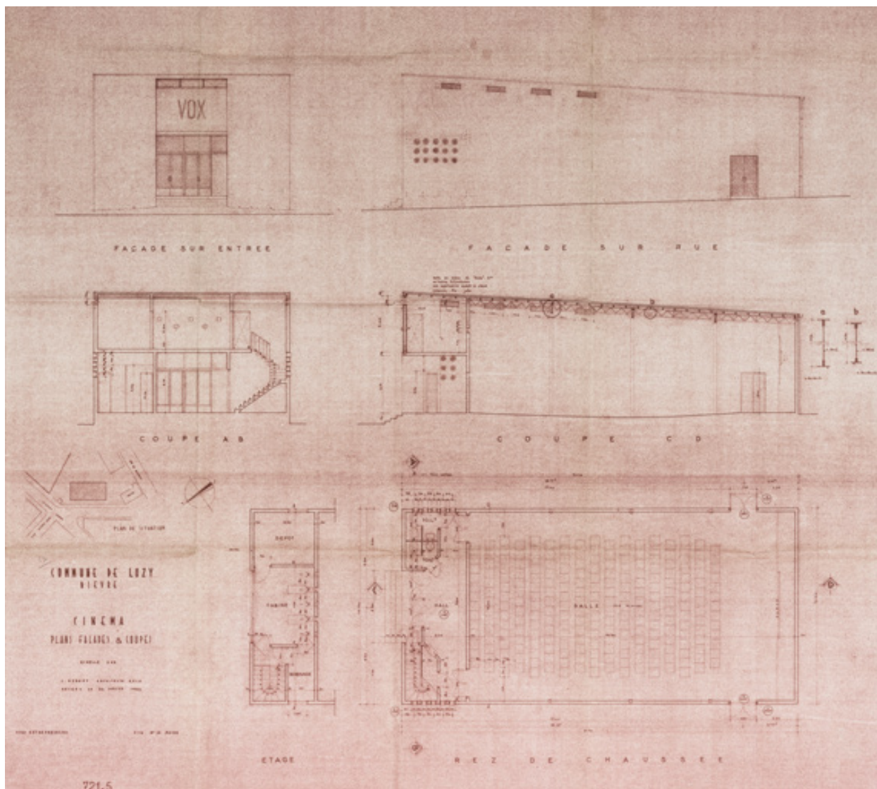
Commune de Luzy. Nièvre. Cinéma. Plans, façades et coupes. 30 janvier 1954.
