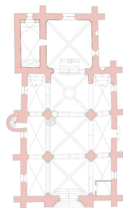
Plan de l'église.
