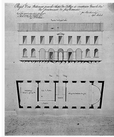
Plan et élévation du bâtiment annexe construit après 1828. Phot. Yves Sancey, Phot. Auguste Robert IVR43_19833900713V
