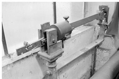
Le mécanisme de pesée. Phot. Jérôme Mongreville IVR43_20022500478X
