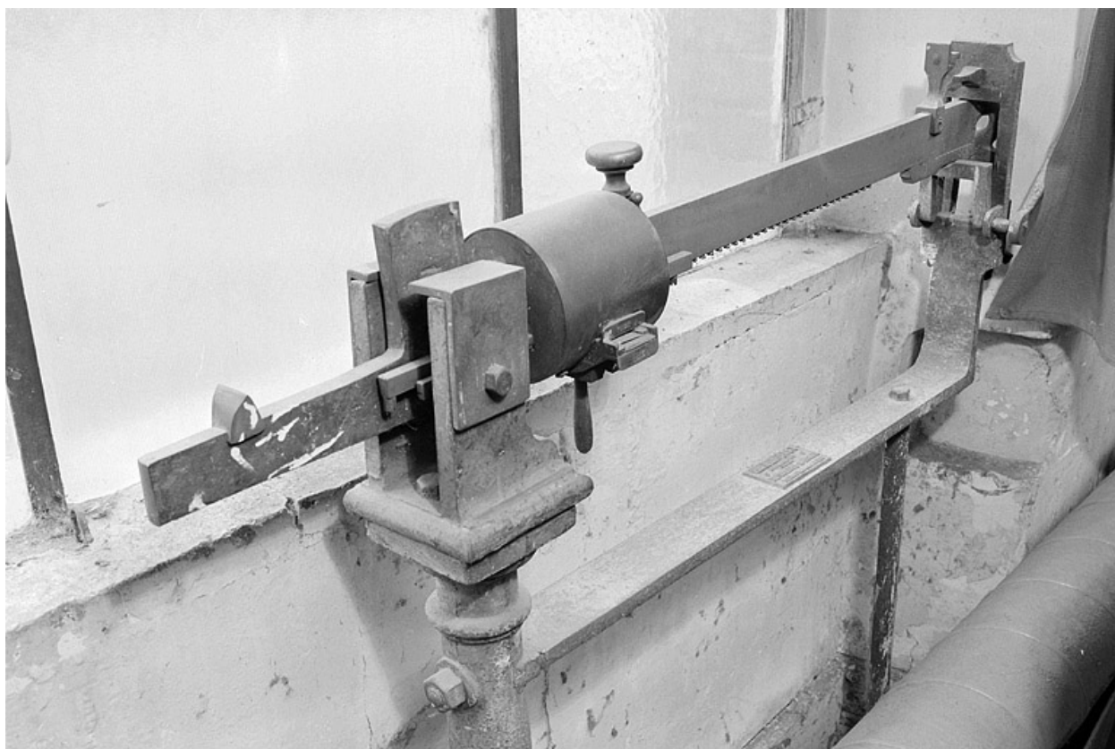
Le mécanisme de pesée.
