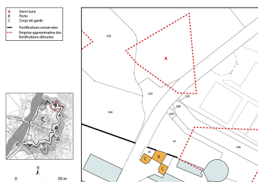
Plan-masse et de situation. Extrait du plan cadastral, 2023, 1/1 000. Dess. Aline Thomas IVR26_20232100171NUDA
