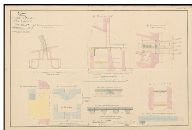
Projet pour 1828 : pont levis pour la Porte Royale. 1828. Autr. auteur inconnu IVR26_20232100137NUC4A
