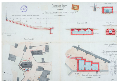
Aménagement d'une citerne à Aisey (1887). Phot. Jérôme Mongreville, Autr. Charles Desgranges IVR43_20167000967NUC4A
