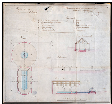
Projet d'une fontaine à Aisey (1830). Phot. Jérôme Mongreville, Autr. auteur inconnu IVR43_20167000942NUC4A
