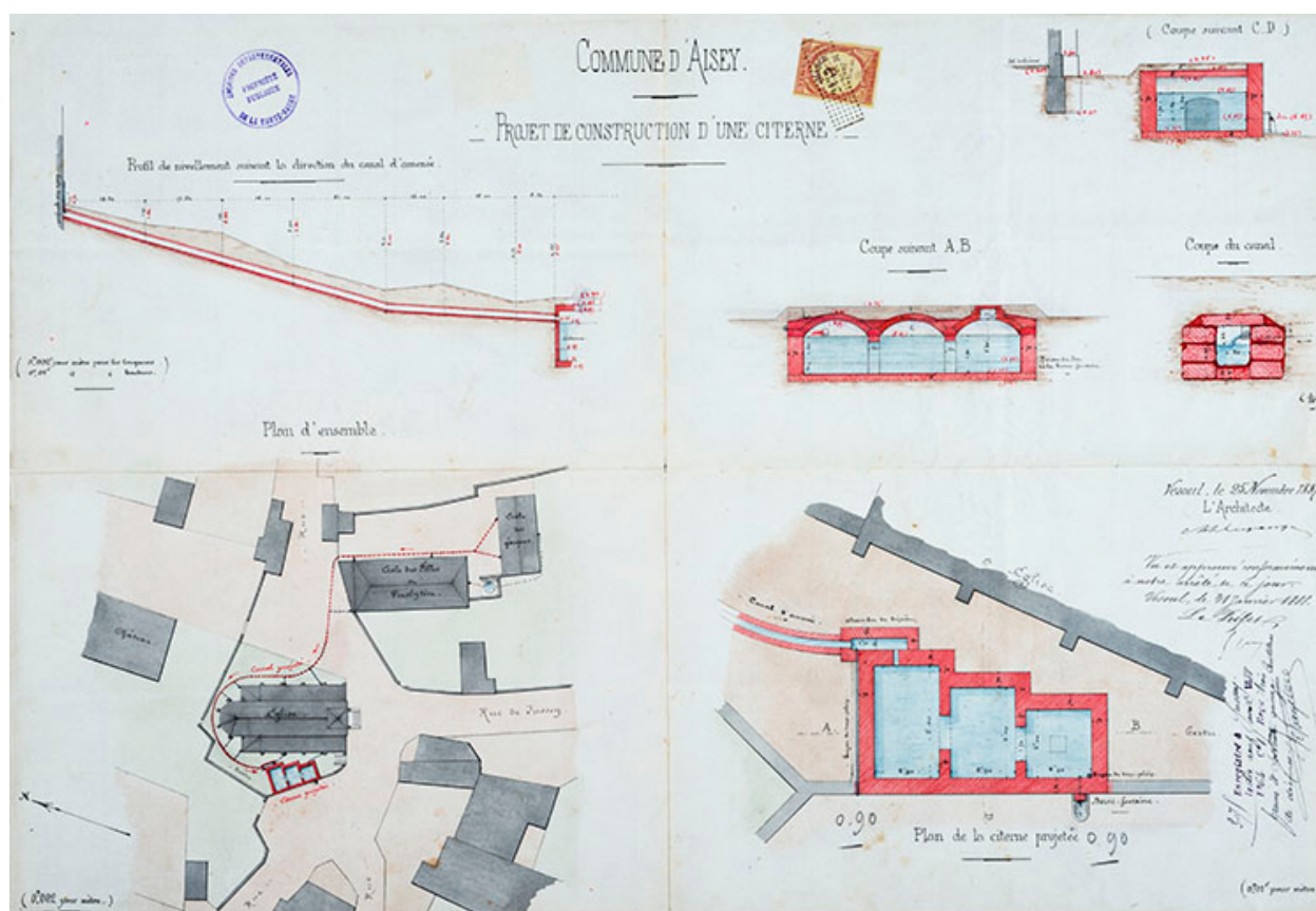
Aménagement d'une citerne à Aisey (1887).
