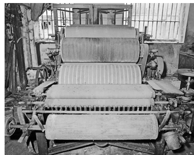
Face arrière. Rouleau en bois, guide-fils, manchons frotteurs, cylindre volant et cylindres travailleurs. Phot. Yves Sancey IVR43_19943901531X
