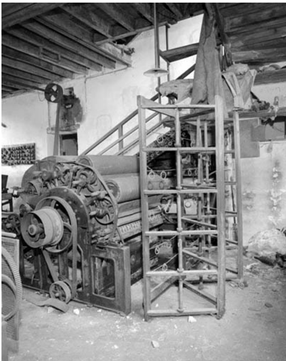
Face avant vue de trois quarts gauche. De droite à gauche, rateliers, guide-fils, carde et ses cylindres travailleurs.
