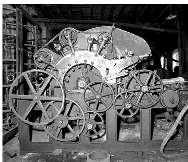
Face latérale droite. Phot. Yves Sancey IVR43_19943901533X
