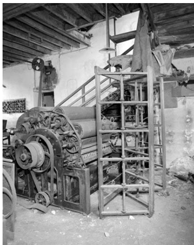
Face avant vue de trois quarts gauche. De droite à gauche, rateliers, guide-fils, carde et ses cylindres travailleurs. Phot. Yves Sancey IVR43_19943901530X
