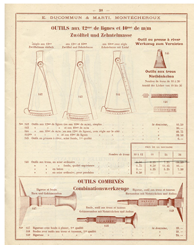
Tarif-album [...] E. Ducommun & Marti successeurs [catalogue de production, p. 21 : outils aux 12e et aux 10e, et outils combinés], [années 1920-1930]. IVR43_20192500995NUC4A
