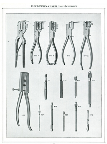
Tarif album n° 5. Fabrique d'outils E. Ducommun & Marti [catalogue de production, p. 48 : pinces aux yeux de ressorts et pinces à morille], [milieu 20e siècle]. IVR43_20192501013NUC4A
