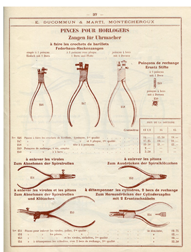
Tarif-album [...] E. Ducommun & Marti successeurs [catalogue de production, p. 37 : pinces pour horlogers], [années 1920-1930]. IVR43_20192500998NUC4A
