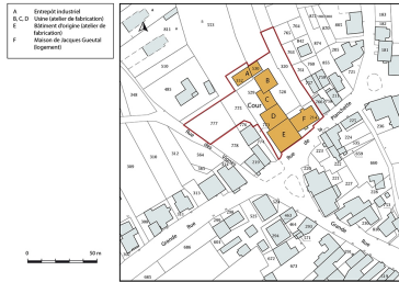
Plan-masse et de situation. Extrait du plan cadastral, 2019, section D. Dess. Bertrand Turina IVR43_20202500303NUDA
