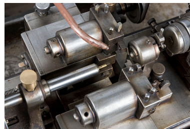
Vue plongeante rapprochée de la partie travaillante, avec la mèche à gauche et les burins au centre.
