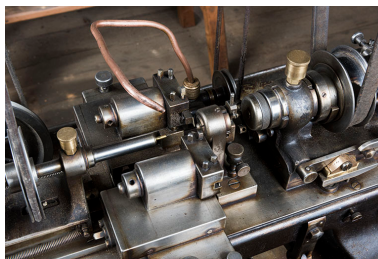
Vue plongeante sur la partie travaillante, avec la mèche à gauche et le burin de coupe au centre.
