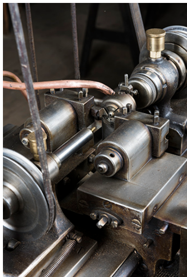
Partie travaillante : mèche à gauche, les deux burins au centre, en avant du support de barre.
