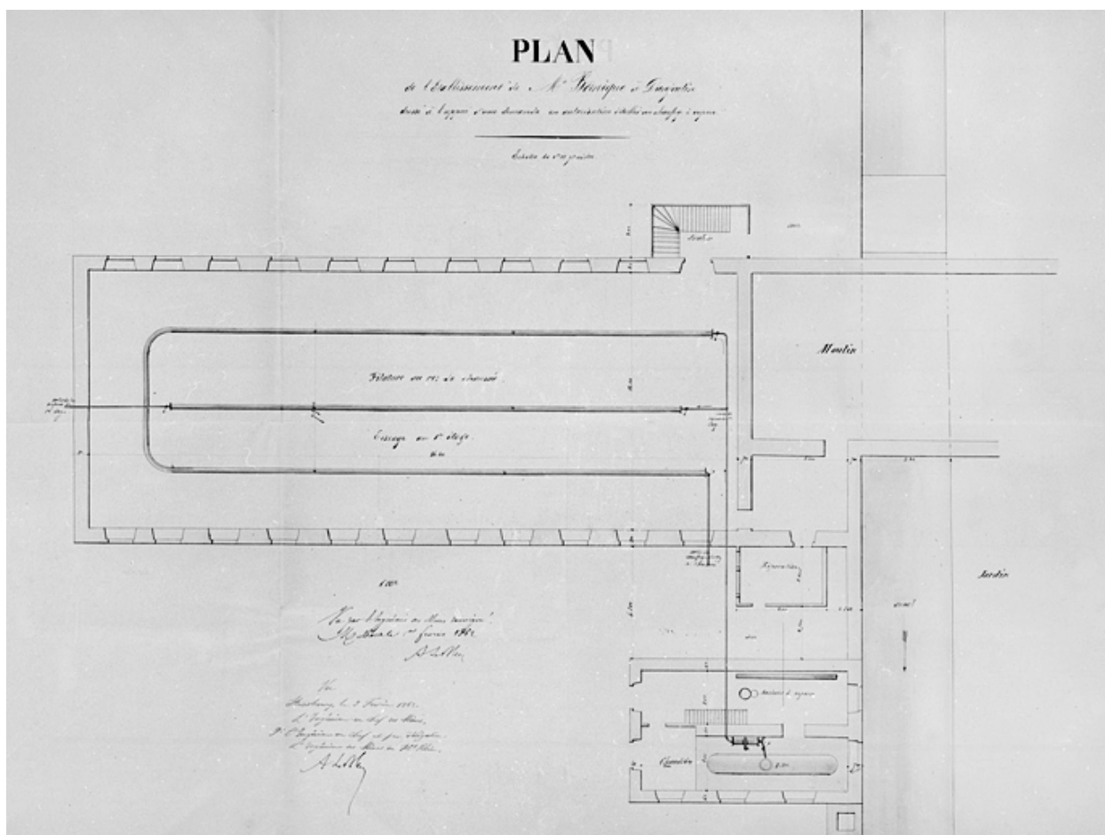
Plan de l'établissement de M. Bornèque à Danjoutin dressé à l'appui d'une demande en autorisation d'établir un chauffage à vapeur.
