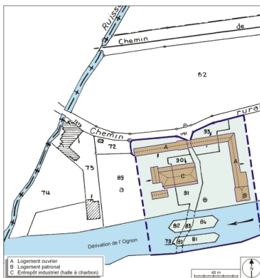
Plan-masse et de situation. Extrait du plan cadastral numérisé, 2005, section A, 1:2000 agrandi à 1:1500. Dess. André Céréza IVR43_20067000063NUDA
