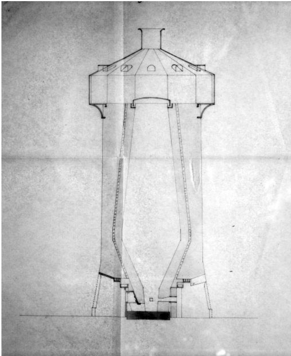
Coupe d'un haut-fourneau au coke.
