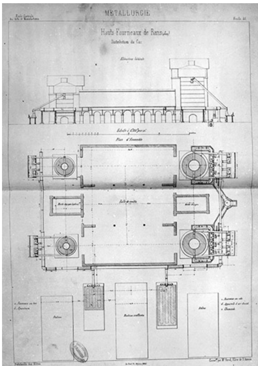
Hauts-Fourneaux de Rans (Jura). Distribution du gaz.
