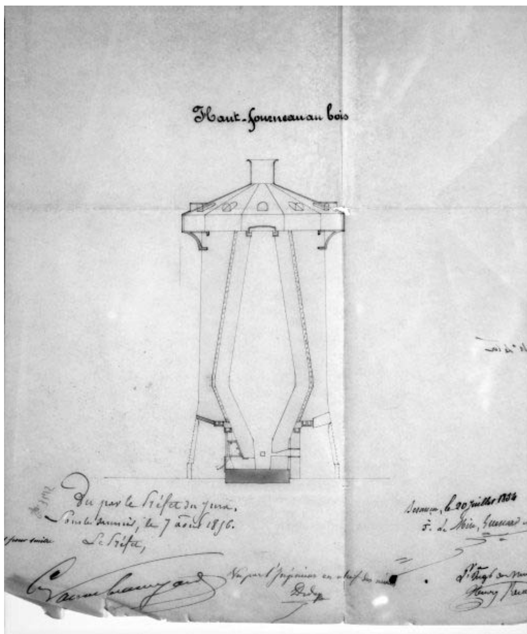
Coupe d'un haut-fourneau au bois.
