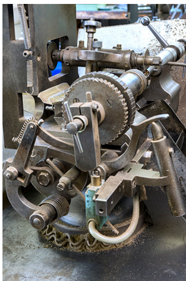
Machine à refendre les morilles : détail du système de commande (avec la fraise à refendre au second plan). Phot. Sonia Dourlot IVR43_20172500474NUC4A
