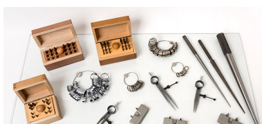
Production de la société Grandidier : jeux de fraises, triboulets, baguiers, compas et clés à ouvrir les fonds de boîte de montre. Phot. Sonia Dourlot IVR43_20172500478NUC4A
