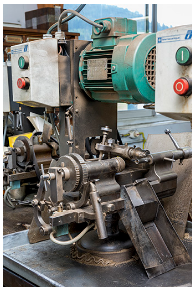
Machine à refendre les morilles (têtes de mandrin). Phot. Sonia Dourlot IVR43_20172500473NUC4A
