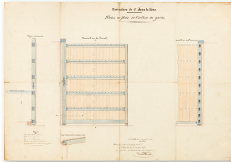
Portes en fonte de l'écluse de garde. Dessin daté du 28 mai 1847. Phot. Thierry Kuntz, Autr. François Anus IVR26_20197100703NUC4A
