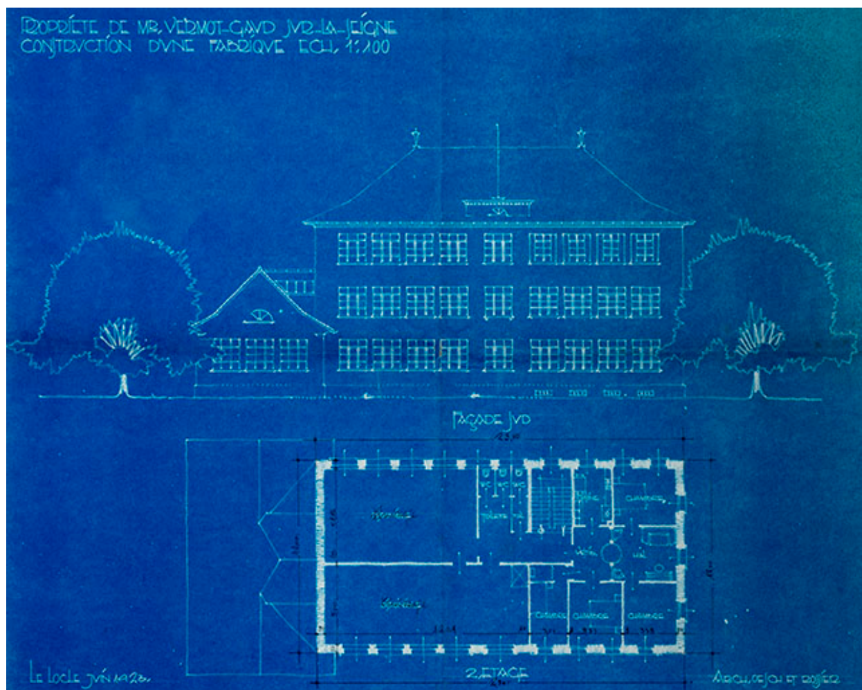
Propriété de Mr Vermot-Gaud, Sur-la-Seigne. Projet de fabrique. Façade sud [et] 2e étage [plan], juin 1923.
