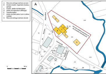
Plan-masse et de situation. Extrait du plan cadastral, 2017, section AD, 1/1 000. Dess. Bertrand Turina IVR43_20182501319NUDA
