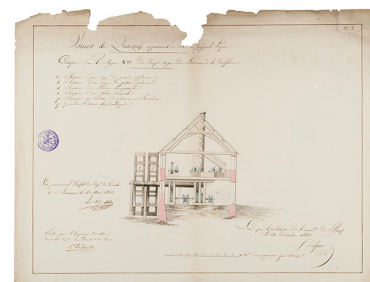
Usines de Quingey [...]. Coupe sur la ligne NO des deux étages du bâtiment de la tréfilerie [...], 1822.
