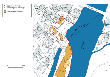
Plan-masse et de situation. Extrait du plan cadastral, 2019. Dess. Bertrand Turina
