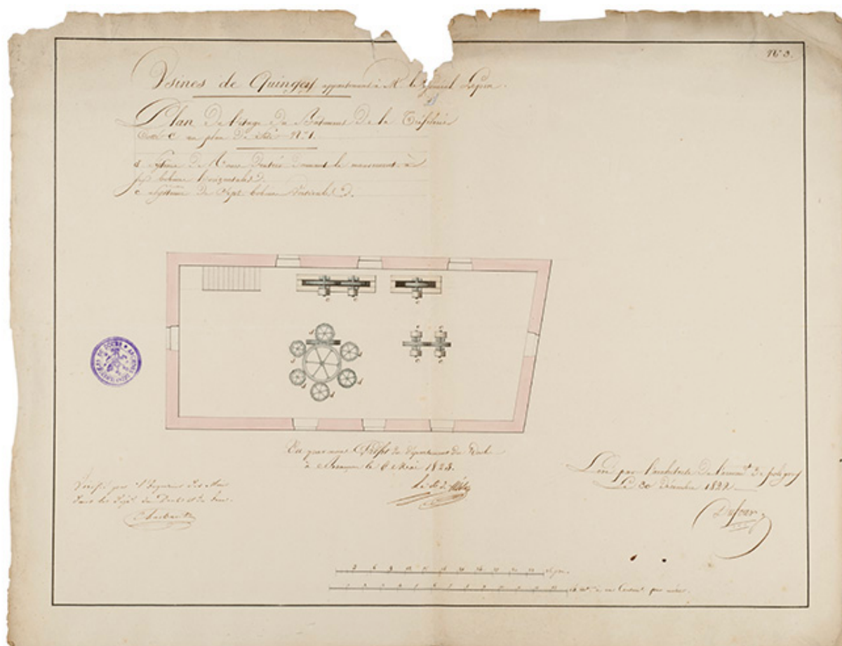
Usines de Quingey [...]. Plan de l'étage du bâtiment de la tréfilerie [...], 1822.
