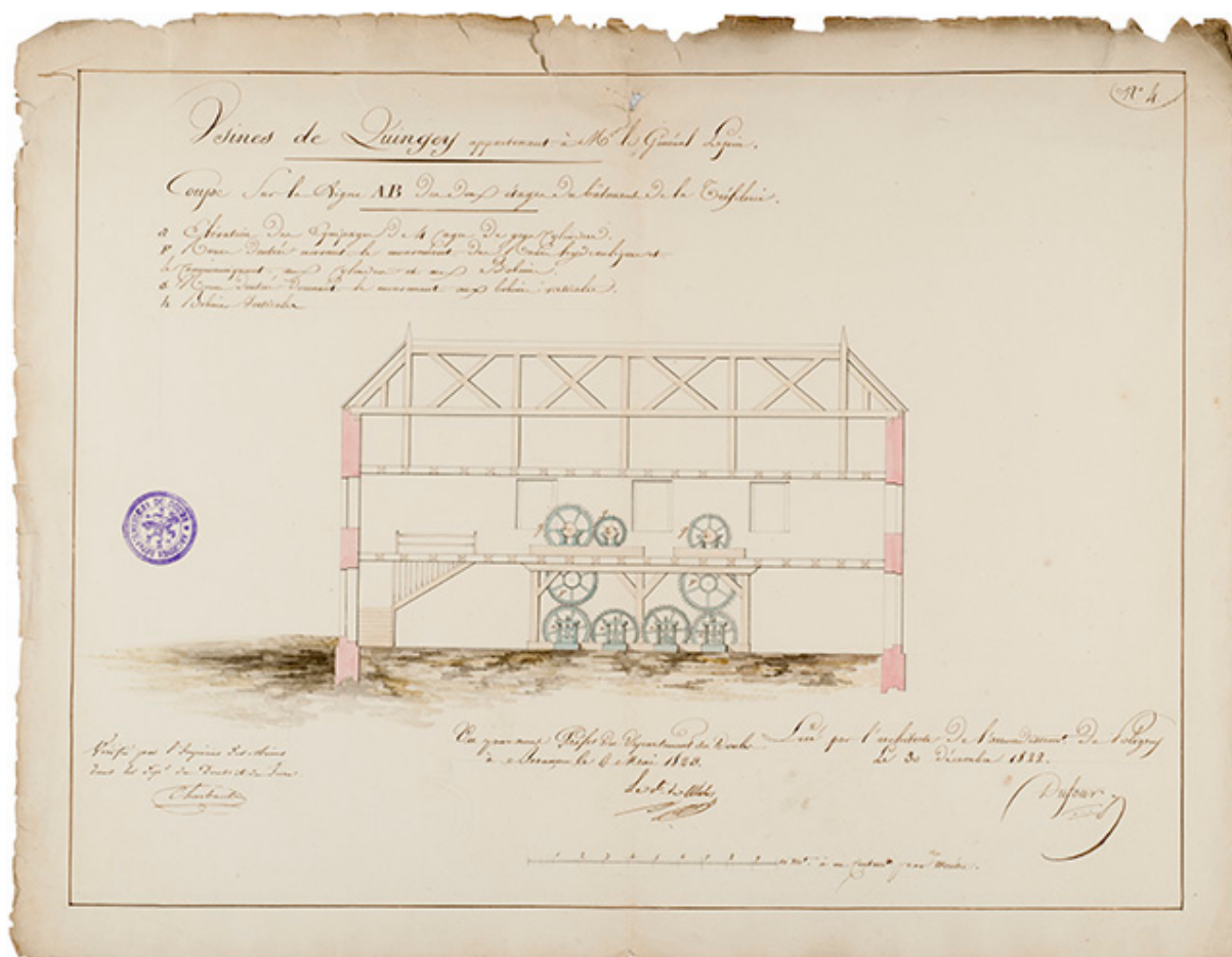
Usines de Quingey [...]. Coupe sur la ligne AB des deux étages du bâtiment de la tréfilerie [...], 1822.
