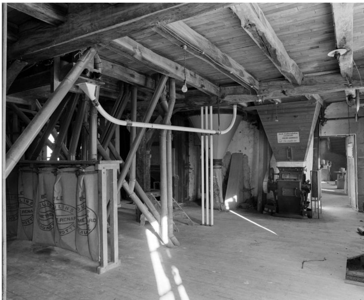
1er étage. Broyeur et ensacheur.
