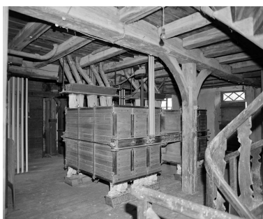
2e étage. Plansichter (Socam, Paris). Phot. Jean-Luc Duthu IVR26_20062106737X
