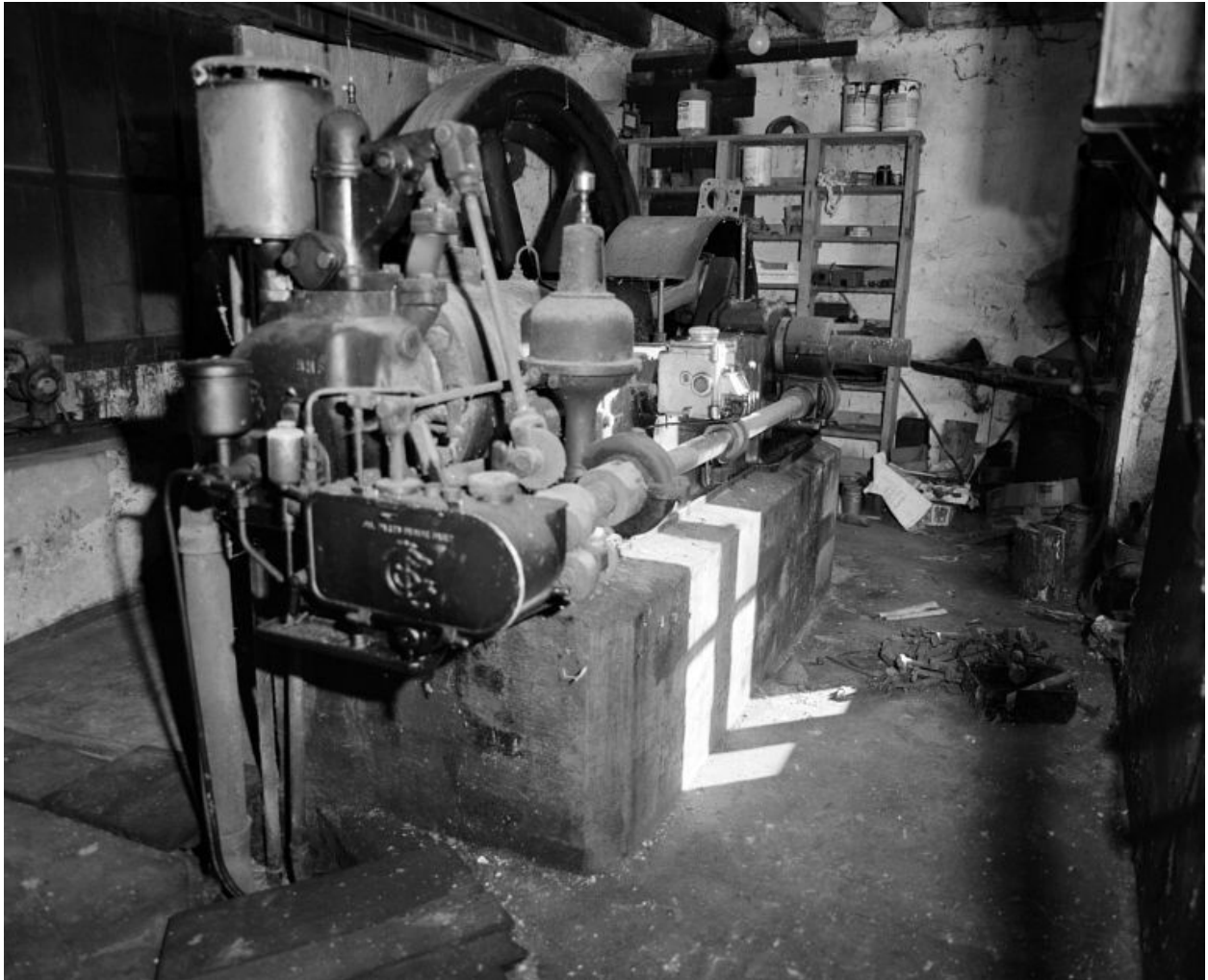
Rez-de-chaussée. Moteur diesel (L. Gardner, constructeur à Patricroft, Angleterre).
