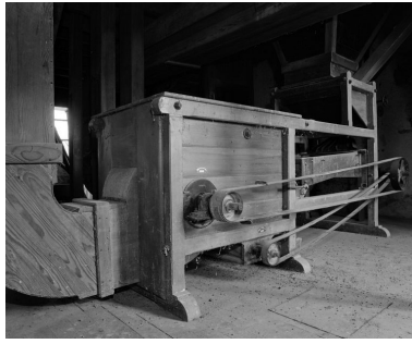
2e étage. Trieur à blé (anciens établissements Lhuillier, Dijon). Phot. Jean-Luc Duthu IVR26_20062106719X
