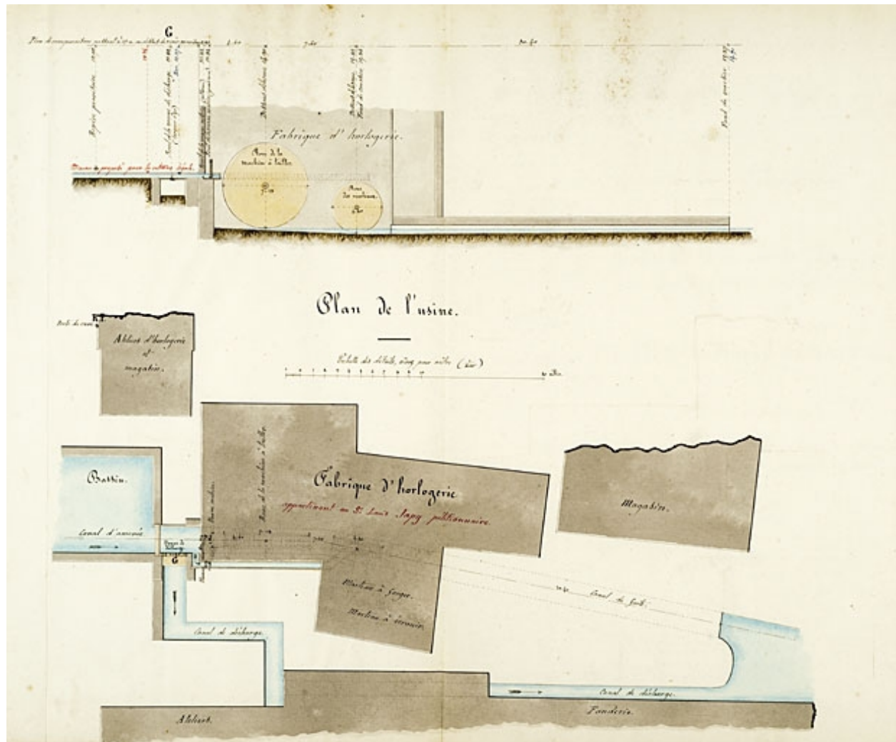
Règlement d'eau de l'usine du sieur Louis Japy située dans le hameau de Berne [Plan de l'usine]. Plan (plume, lavis), coul., 1858, échelle 1/125.
