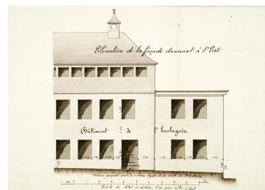
Règlement d'eau de l'usine du sieur Louis Japy située dans le hameau de Berne [Elévation de la façade donnant à l'est]. Plan (plume, lavis), coul., 1858, échelle 1/125. Phot. Jérôme Mongreville IVR43_20112500309NUC4A
