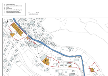
Plan-masse et de situation. Dess. Mathias Papigny IVR43_20132502624NUDA
