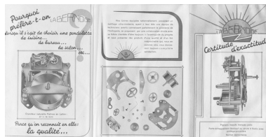
Mouvement d'horlogerie. Dessin, document publicitaire la Bernoise, s.d. [vers 1930]. Phot. Raphaël Favereaux, Autr. IVR43_20122501616NUC2
