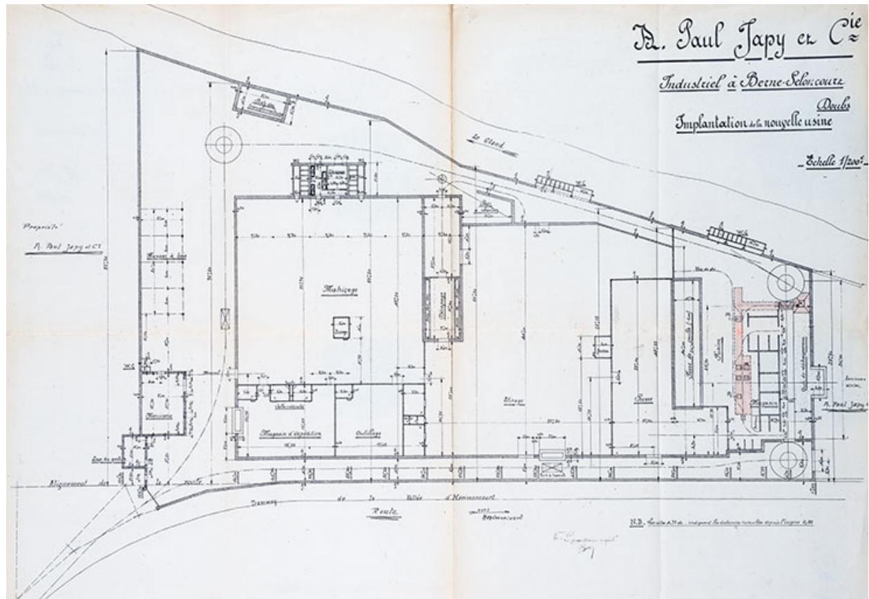
Plan de détail de la nouvelle usine Paul Japy et Cie, industriel à Berne, Seloncourt, tirage, 1/200, s.d. [1920]
