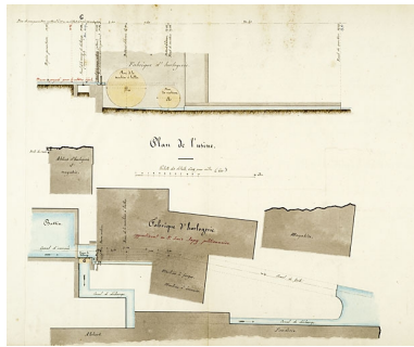
Règlement d'eau de l'usine du sieur Louis Japy située dans le hameau de Berne [Plan de l'usine]. Plan (plume, lavis), coul., 1858, échelle 1/125.
