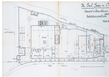
Plan de détail de la nouvelle usine Paul Japy et Cie, industriel à Berne, Seloncourt, tirage, 1/200, s.d. [1920] Phot. Jérôme Mongreville IVR43_20132500515NUC4A
