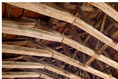
Détail de l'assemblage de la charpente. Phot. Sonia Dourlot IVR43_20157000337NUC2A
