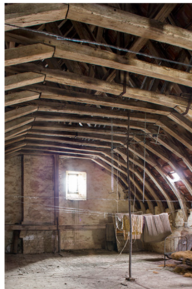
Vue rapprochée de la charpente. Phot. Sonia Dourlot IVR43_20157000336NUC2A
