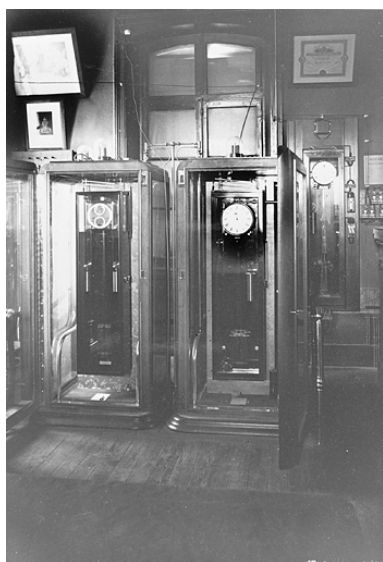
[Vue d'ensemble de deux armoires à température contrôlée], 1924. Phot. Yves Sancey IVR43_20042500108X
