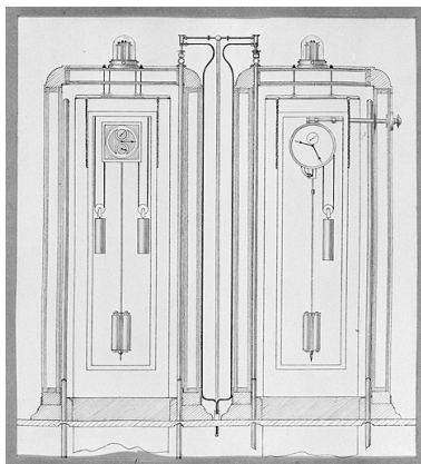
[Coupe de deux armoires à température contrôlée], limite 19e siècle 20e siècle. Dessin incorporé dans un tableau intitulé "Observatoire National de Besançon" et présenté à une exposition à Nancy en 1909. Phot. Yves Sancey IVR43_20042500199X
