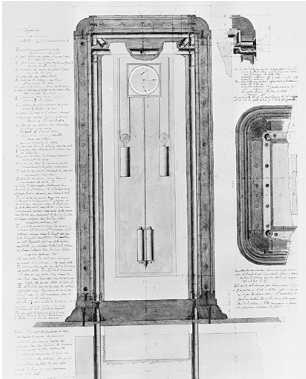
[Coupe d'une armoire à température contrôlée, contenant une pendule], limite 19e siècle 20e siècle.
