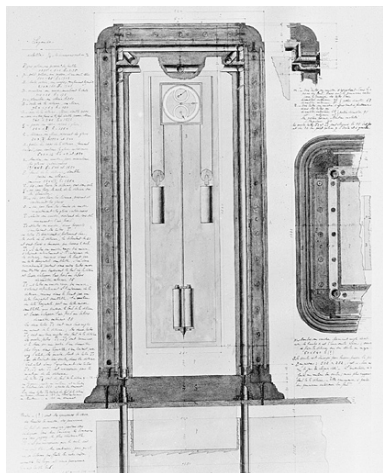
[Coupe d'une armoire à température contrôlée, contenant une pendule], limite 19e siècle 20e siècle. Phot. Yves Sancey IVR43_20042500110X
