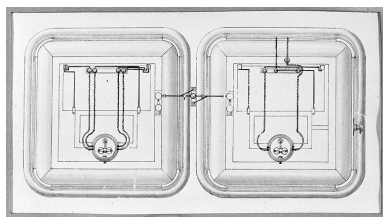
[Dessin de la partie supérieure de deux armoires à température contrôlée, montrant les relais et leur câblage], limite 19e siècle 20e siècle. Dessin incorporé dans un tableau intitulé "Observatoire National de Besançon" et présenté à une exposition à Nancy en 1909. Phot. Yves Sancey IVR43_20042500200X
