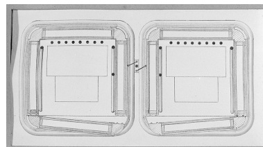
[Plan de deux armoires à température contrôlée], limite 19e siècle 20e siècle. Dessin incorporé dans un tableau intitulé "Observatoire National de Besançon" et présenté à une exposition à Nancy en 1909. Phot. Yves Sancey IVR43_20042500201X
