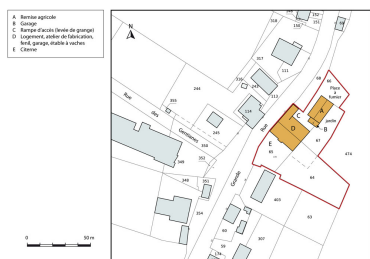
Plan-masse et de situation. Extrait du plan cadastral, 2013, section AC. Dess. Mathias Papigny IVR43_20142501551NUDA
