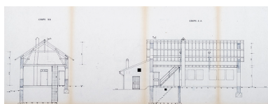
Etat des lieux [coupes], vers 1983. Phot. Sonia Dourlot, Autr. auteur inconnu IVR43_20162501049NUC4A
