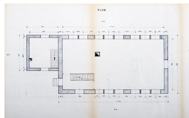
Etat des lieux [plan], vers 1983. Phot. Sonia Dourlot, Autr. auteur inconnu IVR43_20162501050NUC4A
