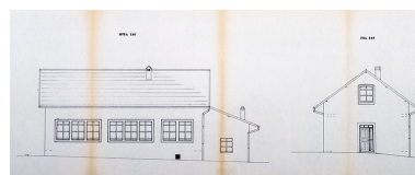
Etat des lieux. Sud Est [et] Nord Est [élévations], vers 1983. Phot. Sonia Dourlot, Autr. auteur inconnu IVR43_20162501047NUC4A
