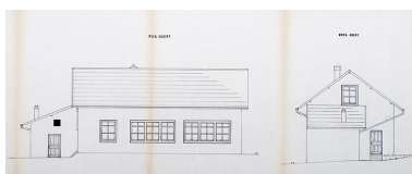
Etat des lieux. Sud Ouest [et] Nord Ouest [élévations], vers 1983. Phot. Sonia Dourlot, Autr. auteur inconnu IVR43_20162501048NUC4A
