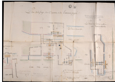
2e feuille de plan des usines de Conflandey [...] Plan et coupe du haut fourneau, plan de la forge, des courants et du laminage projeté. Phot. Daniel Lebé, Autr. Beaujard IVR43_19907000208XA
