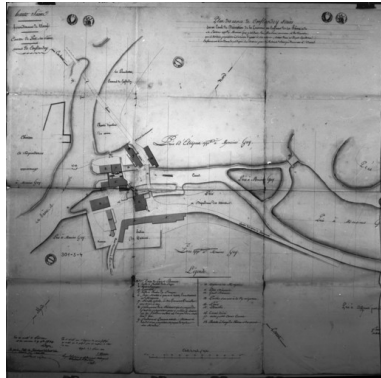
Plan des usines de Conflandey situées sur le canal de dérivation de la Lanterne [...] appartenant à M. Guy [...]. Phot. Yves Sancey, Autr. Beaujard IVR43_19877000029X
