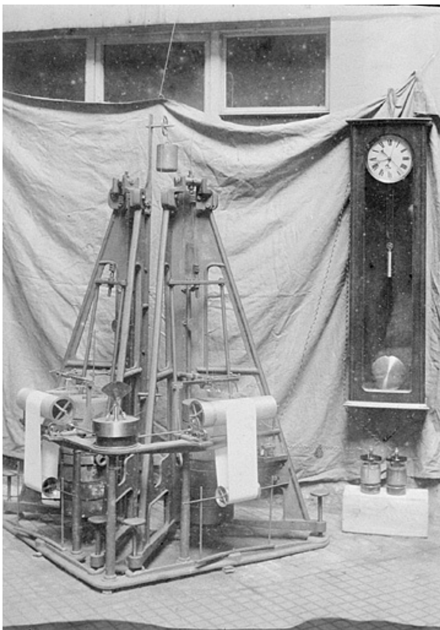
[Sismographe et pendule], avant 1909. Photographie incorporée dans un tableau intitulé "Observatoire National de Besançon" et présenté à une exposition à Nancy en 1909.
