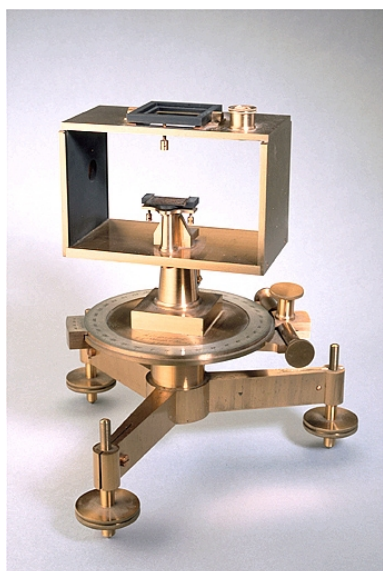
Balance magnétique de Mascart. Phot. Jérôme Mongreville IVR43_20032500834XA
