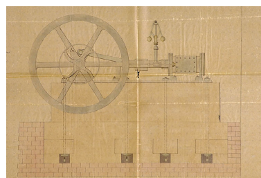
[Elévation de la machine à vapeur]. Phot. Jérôme Mongreville IVR43_20057000564NUCA
