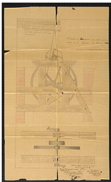
Machine de 3 ch pour extraire les eaux douces à la saline de Melecey. Phot. Jérôme Mongreville IVR43_20057000562NUCA
