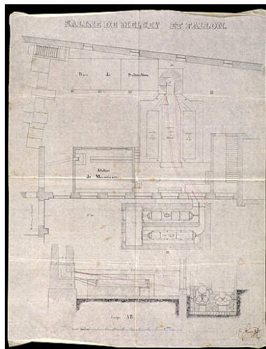
Saline de Melcey et Fallon [plan de la salle des machines]. Phot. Jérôme Mongreville, Phot. Lamare IVR43_20057000560NUCA
