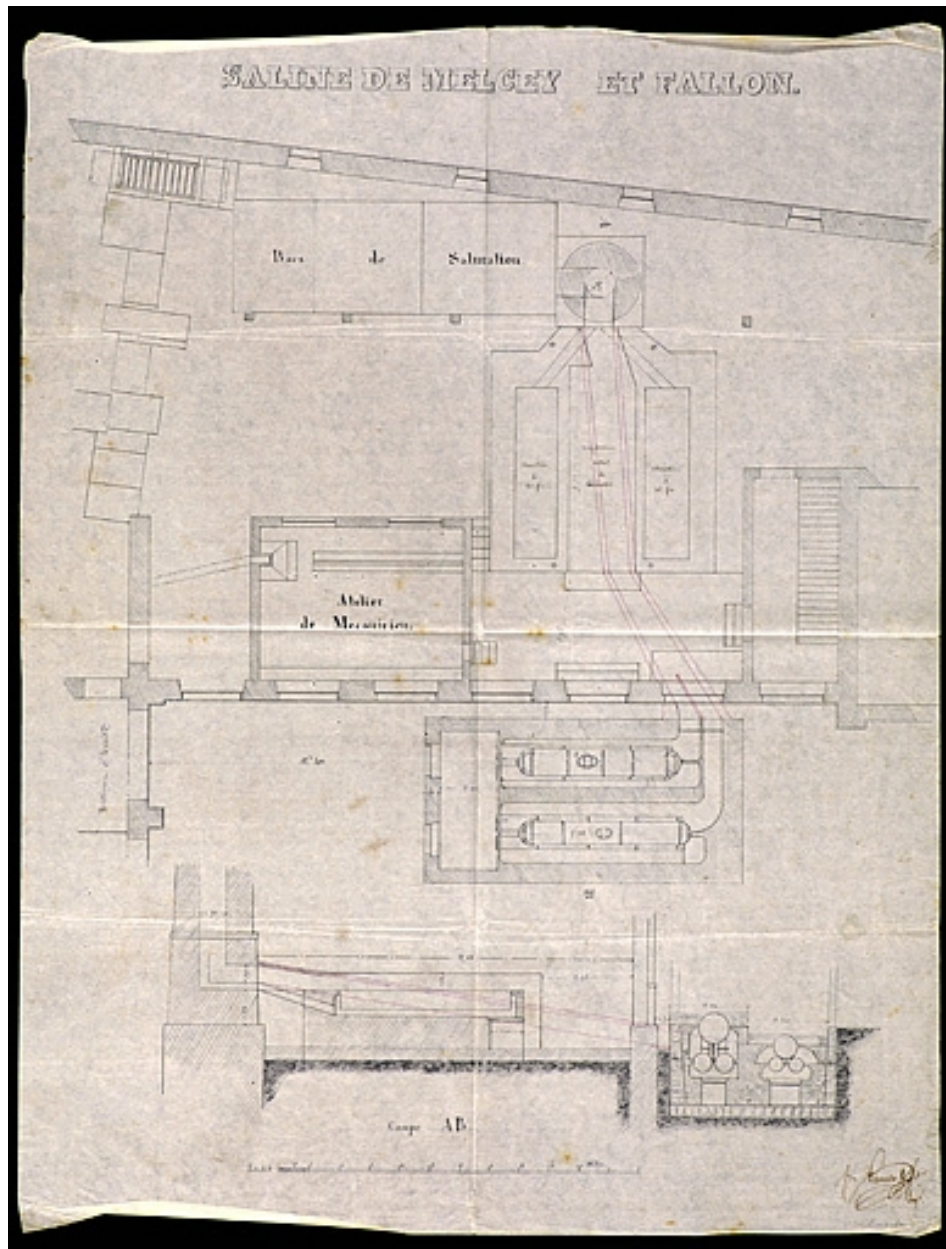
Saline de Melcey et Fallon [plan de la salle des machines].
