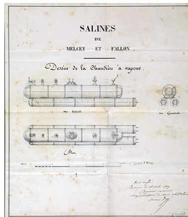
Salines de Melcey et Fallon [dessin de la chaudière à vapeur]. Phot. Jérôme Mongreville, Phot. Lamare IVR43_20057000561NUCA
