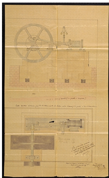
[Elévation et vue en plan de la machine à vapeur]. Phot. Jérôme Mongreville IVR43_20057000563NUCA
