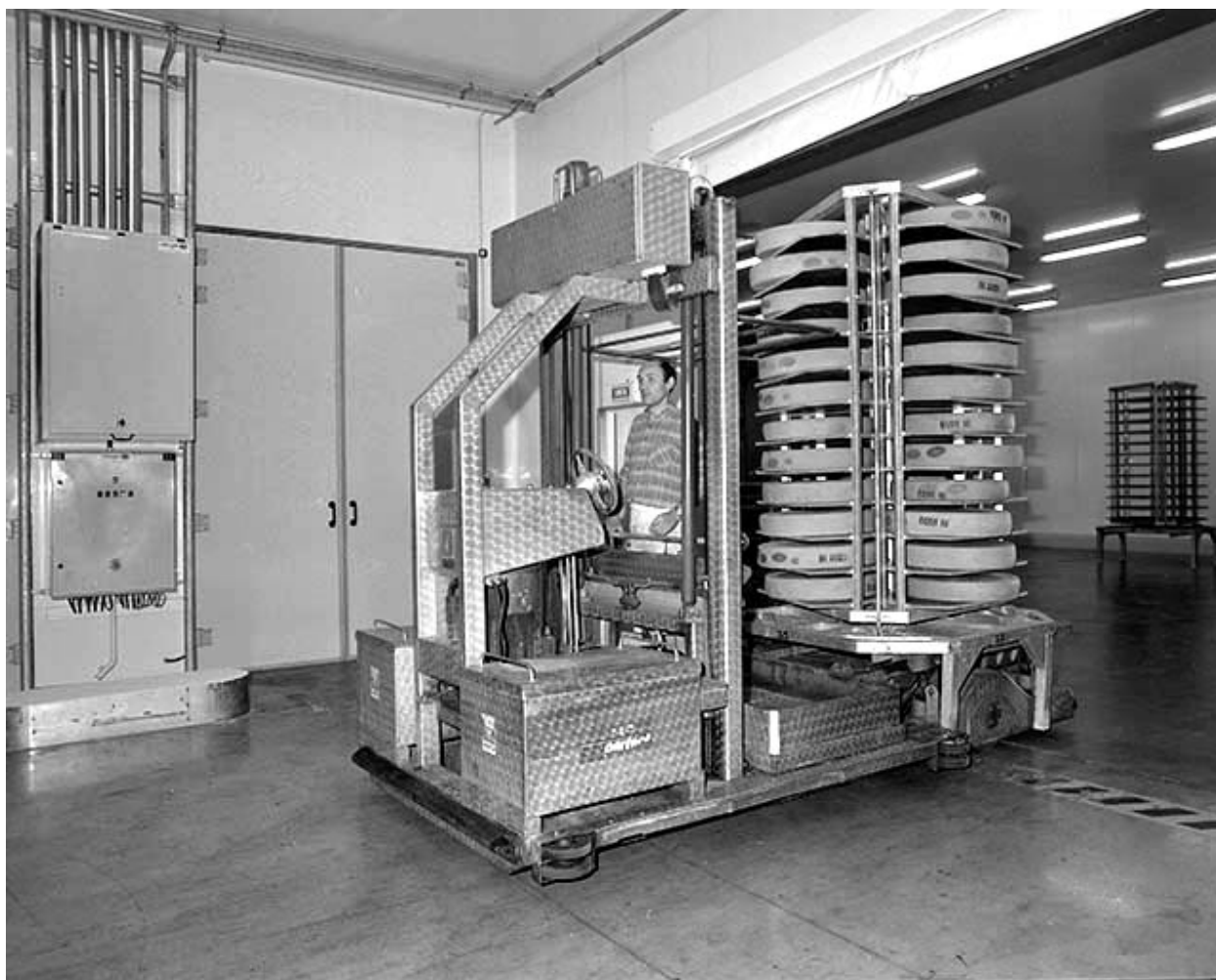
Transport des meules sur chariot électrique.
