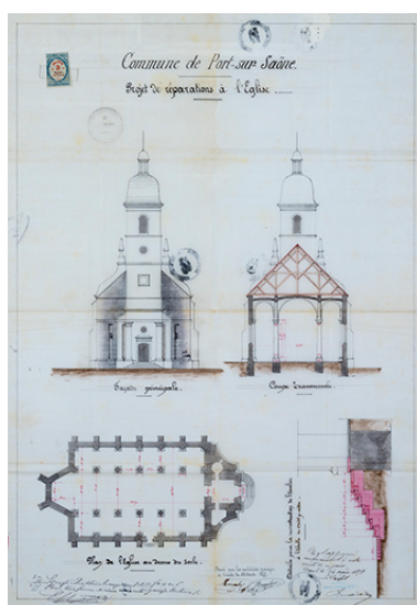
Plan pour projets de réparations, 1877.
