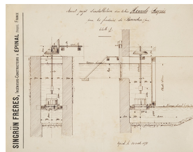
Avant-projet d'installation d'une turbine Hercule-Progrès, Epinal, le 14 octobre 1898. IVR43_20203900156NUC2A
