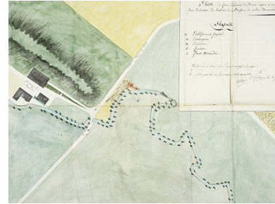
Plan du cours de la rivière de Braine, depuis et compris le fourneau Beaudin [...], le 12 juillet 1811. IVR43_20203900173NUC2A
