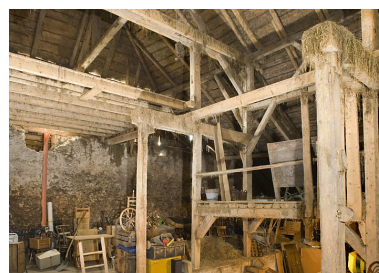
Déchargeuse : charpente et plateforme dans la grange.
