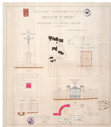
Projet du cimetière (1892). Phot. Jérôme Mongreville, Autr. J.-B. Martin IVR43_20167000953NUC4A
