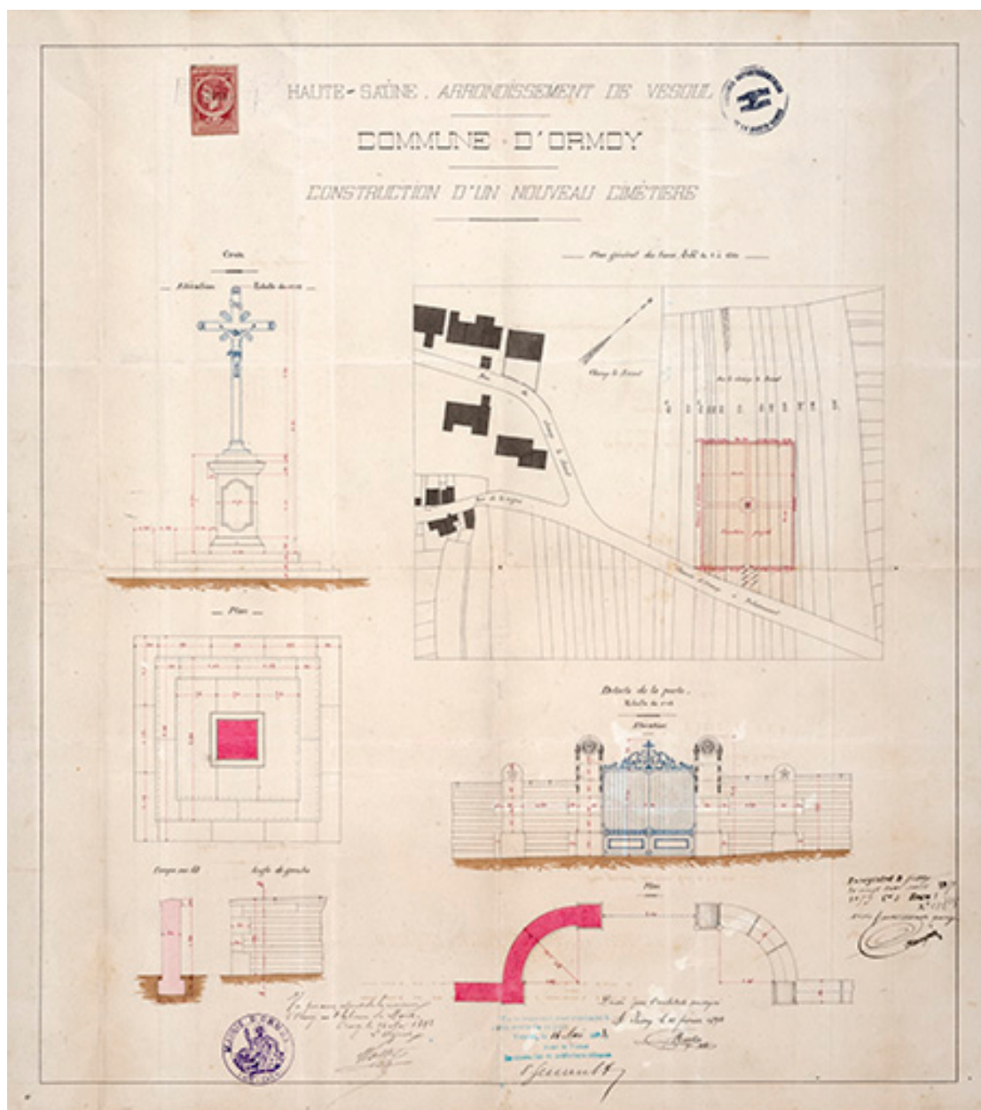
Projet du cimetière (1892).
