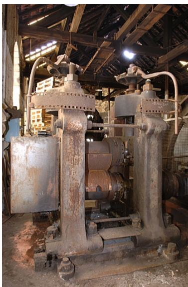
Les cylindres de laminage. Phot. Jérôme Mongreville IVR43_20057000046NUCA
