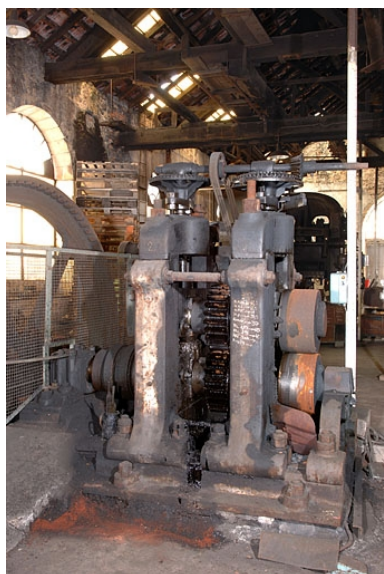
Les cylindres "élargisseurs". Phot. Jérôme Mongreville IVR43_20057000063NUCA
