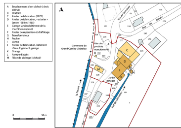
Plan-masse et de situation. Extrait du plan cadastral, 2016, section A, 1/2 500 agrandi à 1/1 000. Dess. Bertrand Turina IVR43_20182501338NUDA
