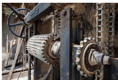
Atelier de fabrication : châssis de scie Socolest, pignon et rouleau. Phot. Sonia Dourlot IVR43_20172501686NUC4A
