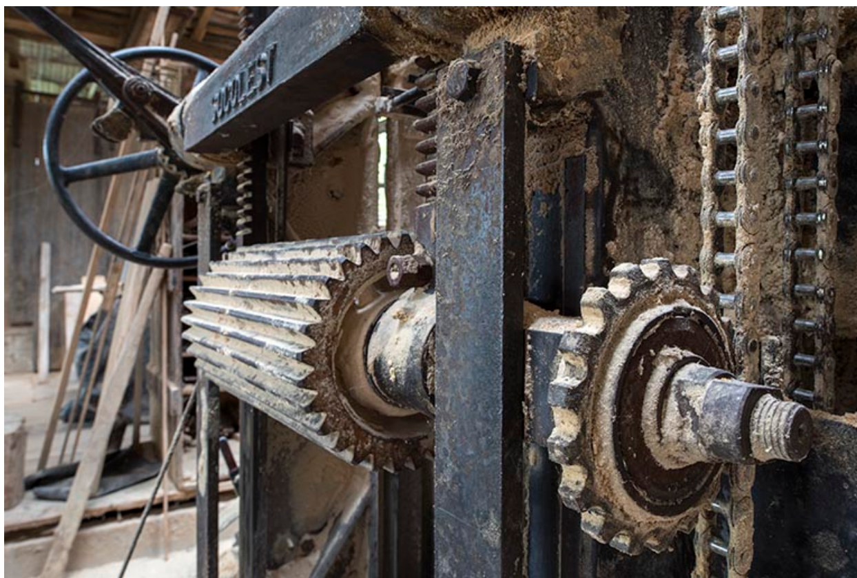
Atelier de fabrication : châssis de scie Socolest, pignon et rouleau.
