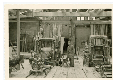
[Sciage au gros châssis de scie Socolest, vu depuis l'entrée de l'atelier], années 1960. Autr. auteur inconnu IVR43_20172501519NUC4A
