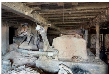
Atelier de fabrication, sciurier : massifs en maçonnerie de la scie Socolest (à gauche) et d'un châssis démonté. Phot. Sonia Dourlot IVR43_20172501698NUC4A
