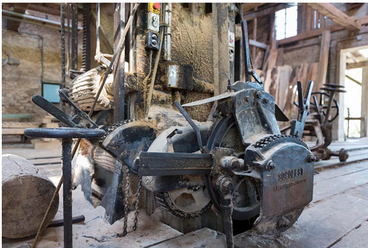
Atelier de fabrication : châssis de scie Socolest, détail du système moteur.
