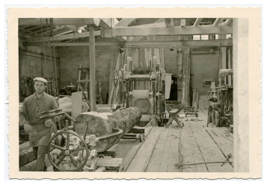
[Sciage au gros châssis de scie Socolest, vu depuis le fond de l'atelier : un tronc d'arbre est approché de la scie], années 1960. Phot. auteur inconnu IVR43_20172501518NUC4A
