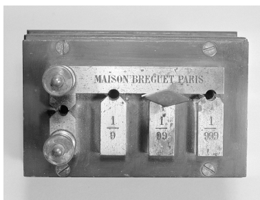
Shunt : face supérieure. Phot. Jérôme Mongreville IVR43_20032500881X
