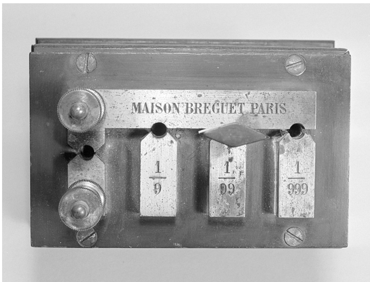
Shunt : face supérieure.
