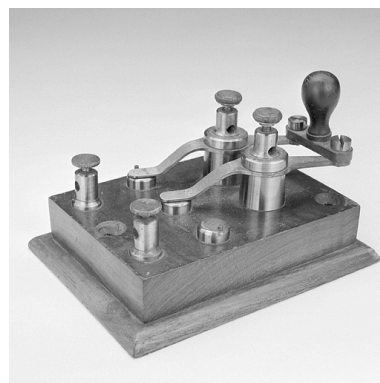
Commutateur. Phot. Jérôme Mongreville IVR43_20032500883X
