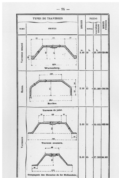
[Coupe de différents modèles de traverses métalliques : Vautherin, Vautherin modifié, Heindl], 1886. Phot. Yves Sancey, Autr. Simon (? Cantagrel IVR43_20083900922NUC2A
