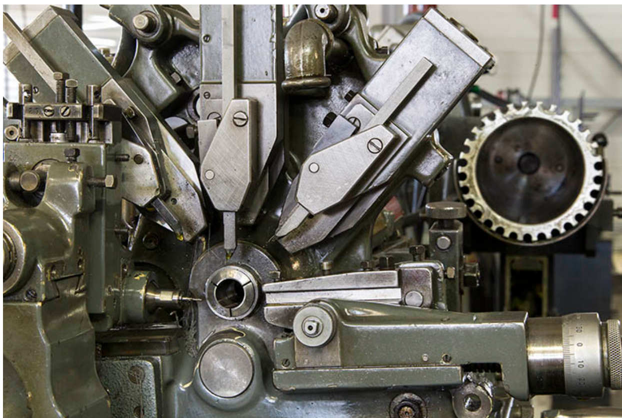
Usine de décolletage Perrenoud (Charquemont). Machine à décolleter Tornos.
