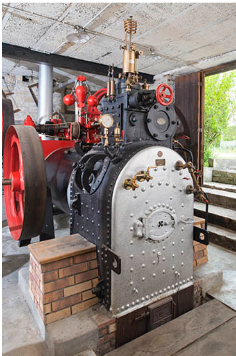
Machine à vapeur de la scierie Lescot (Rémondans-Vaivre).
