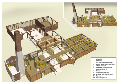
Vue axonométrique de la tuilerie-scierie des Combes de Punay (Malbrans). Dess. Mathias Papigny IVR43_20162501772NUDAQ
