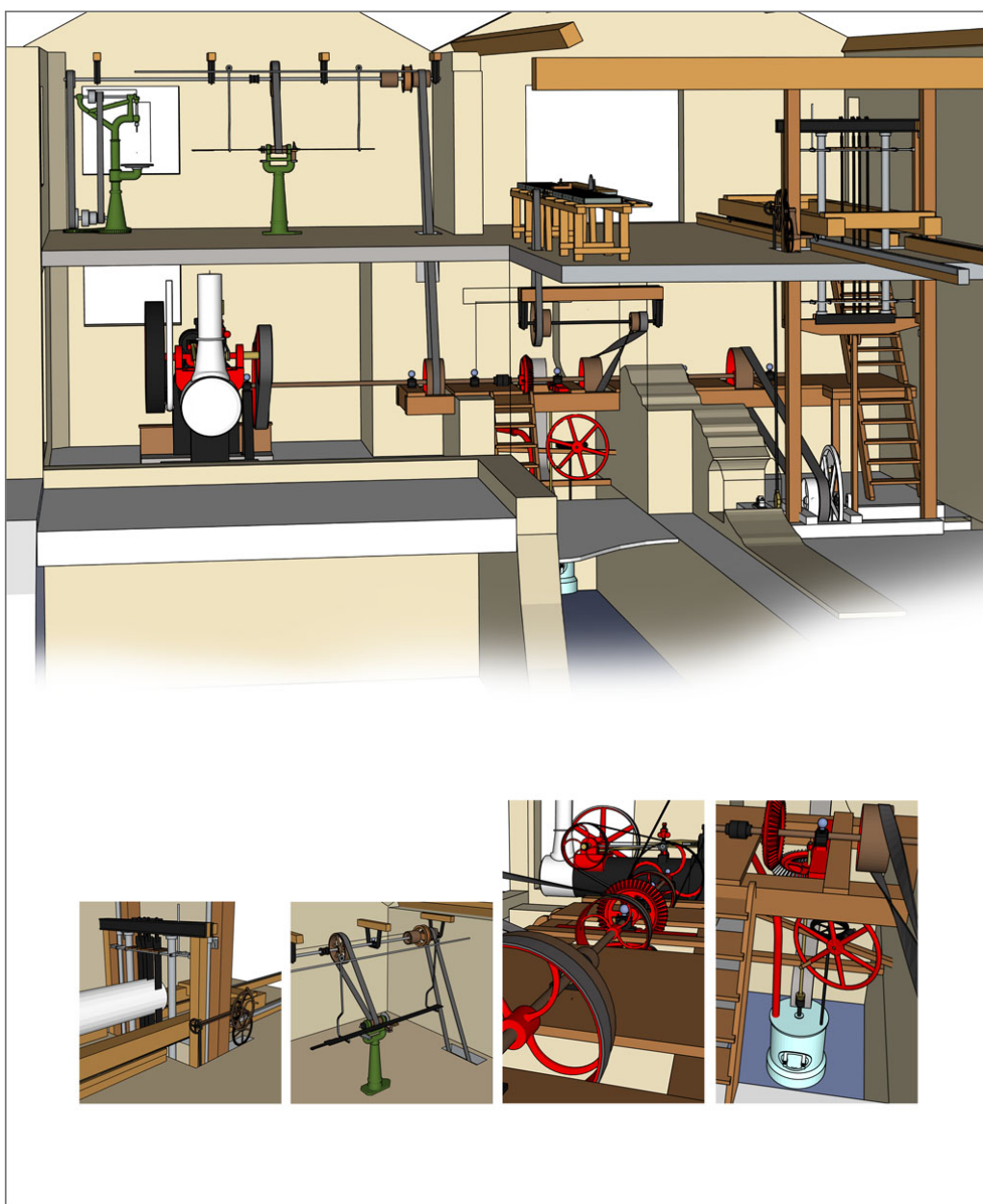
Scierie Lescot à Rémondans-Vaivre. Schéma de distribution de la force motrice.
