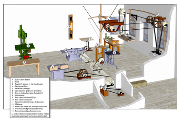
Menuiserie Baudiquey (Sancey- le-Long). Plan de disposition des machines à l'étage de soubassement Dess. Mathias Papigny IVR43_20162501771NUDAQ
