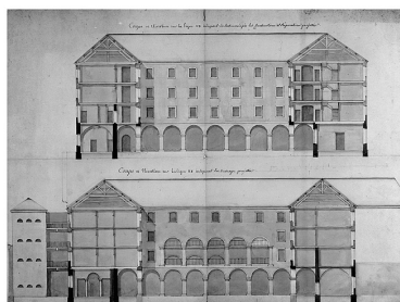
Elévations des façades des bâtiments conventuels après transformation en séminaire (projet de transformation).
